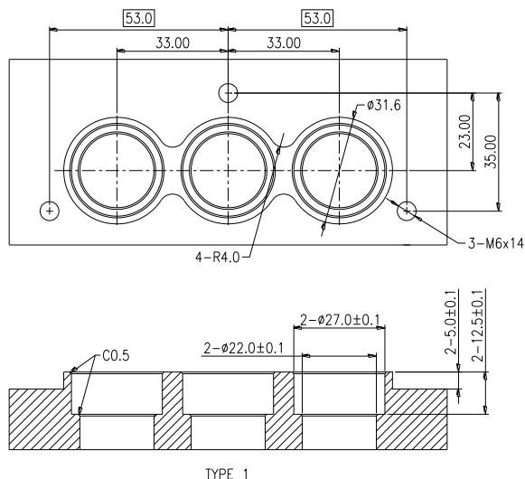
ECT 塑胶 3 孔面板安装尺寸：
