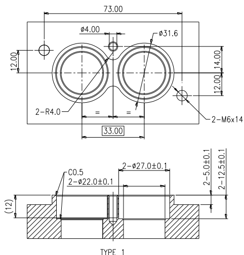
ECT 塑胶 2 孔面板安装尺寸：
