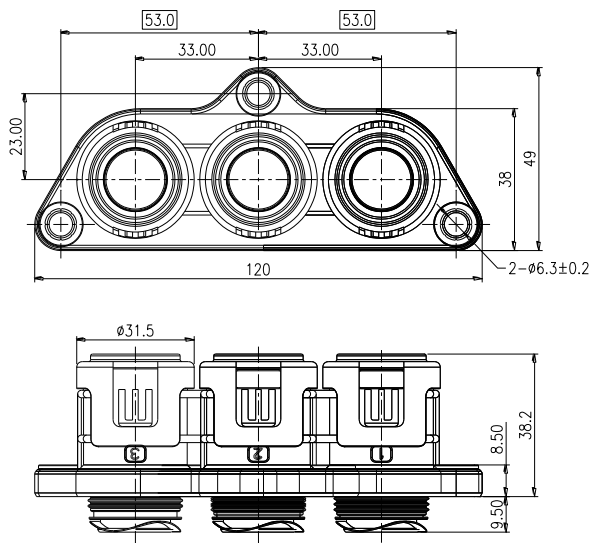
ECT 塑胶 3 孔外形尺寸：
