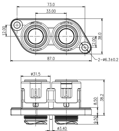
ECT 塑胶 2 孔面板安装尺寸：
